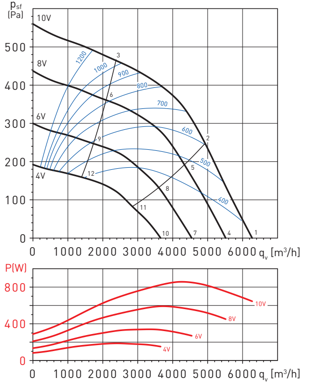
CRHB-450 N ECOWATT
